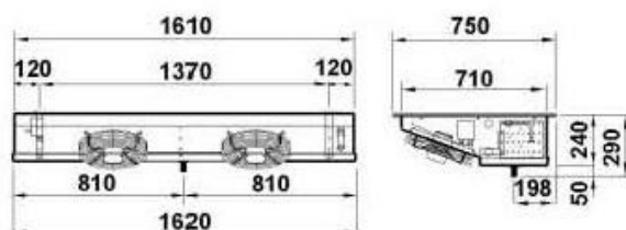
Evaporatore GS340
