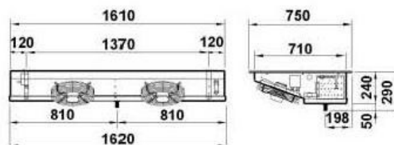
Verdampfer GS340
