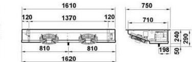
Evaporador GS340
