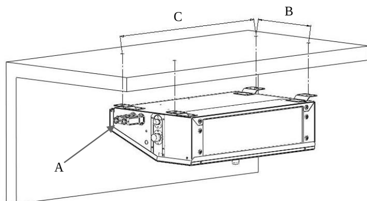
Evaporatore GS340
