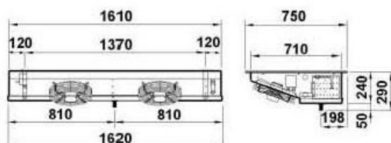
Evaporateur GS340
