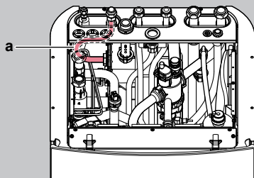
a Hűtőközegvezeték
