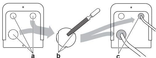
a Kilökölapnyílás b Leélezni c Tömítőanyag, stb.
