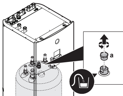
a Tartálynyílás
