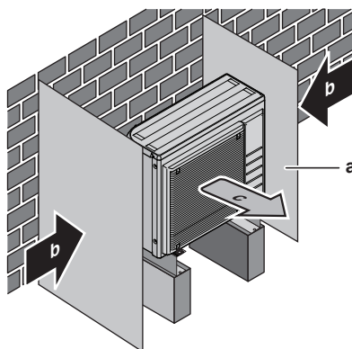
a Terelőlemez b Uralkodó szélirány c Levegőkimenet
