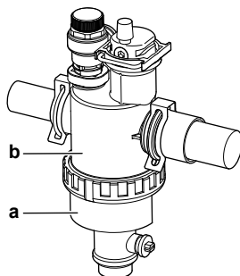
a A kicsavarandó alsó rész b Vízszűrő háza
