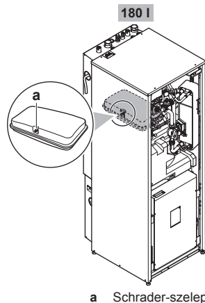
a Schrader-szelep
