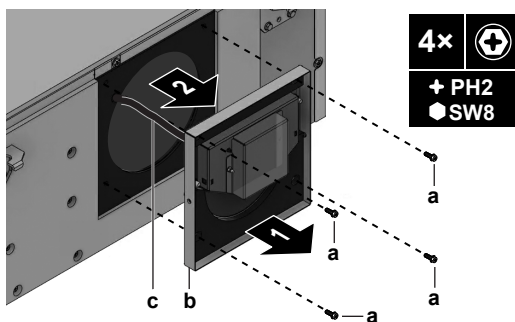
a Csavar b Huzatszabályzó c Huzatszabályozó vezetéke
