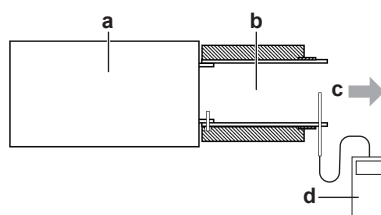
a SV egység b Levegőkimenet légcsatorna c Levegőfúvás iránya d Hődrótos légsebességmérő
