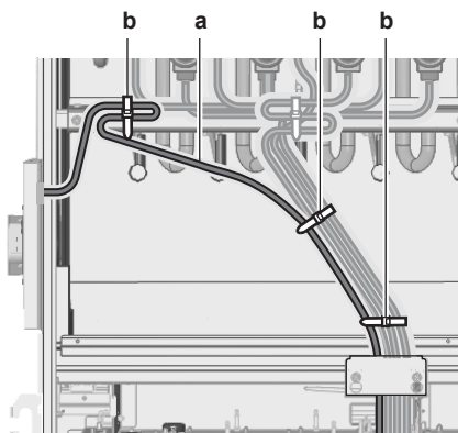
a Huzatszabályozó vezetéke b Kábelszorító
